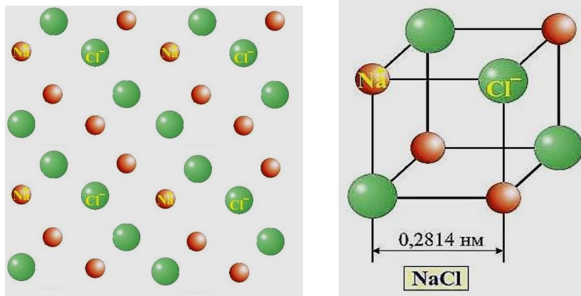
Рис.87. Условное расположение частиц натрия Na и хлора Cl в кристалле
