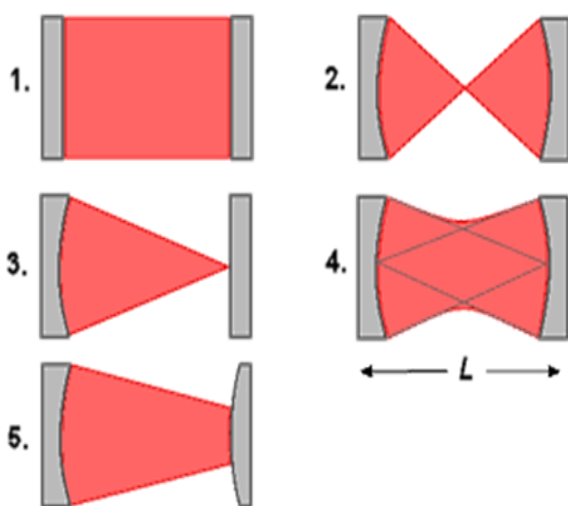
Рис.79. Резонаторы Фабри-Перо:
