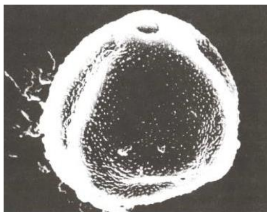
Рис.109. Пример резонатора -фрактальная структура мозгового песка
