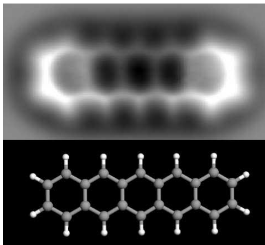
Рис.92. На картинке, полученной с помощью бесконтактной атомно-силовой микроскопии AFM (вверху), можно предположить пять углеродных колец гексагональной формы и визуализировать позиции «атомов» углерода и водорода. На иллюстрации внизу распространенная схема той же молекулы: серые шарики – атомы углерода, белые – водорода.
