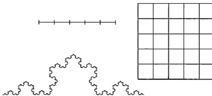
Рис.110. Два вида самоподобия: стандартное и фрактальное
