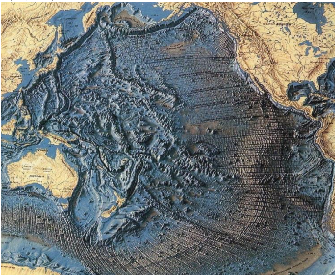
Карта рельефа дна Тихого океана
