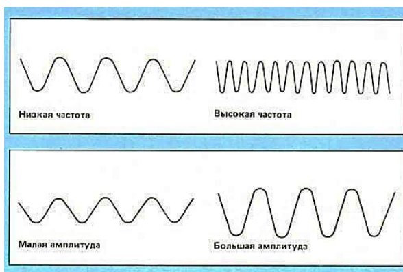
Рис.3. Частота и амплитуда плотности среды в волне
