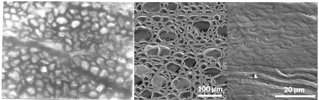
Рис.96. Микроструктура торцовой поверхности древесины
