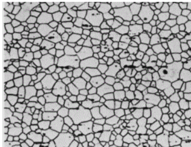
Рис.98. Зернистая структура стали
