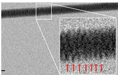
Рис.56. Фотография предполагаемой ДНК (DNA Helix).
