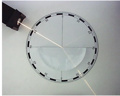
Рис.25. Так отличается истинное положение излучателя А от видимого А 1 при наблюдении из более плотной среды.
