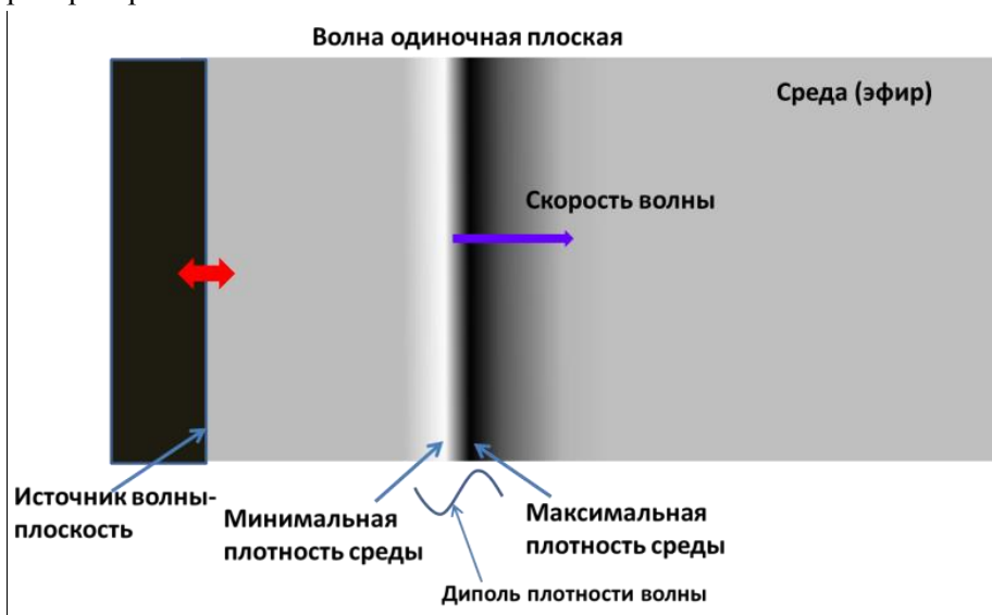
Рис. 13. Плоская одиночная волна
