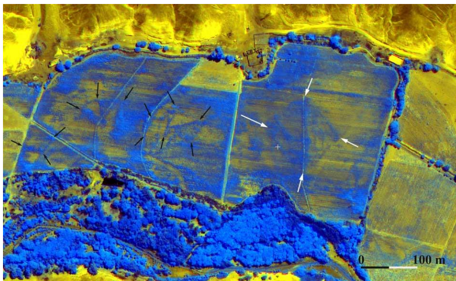
Рис.69. С помощью спутниковых инфракрасных изображений в Египте обнаружено более тысячи гробниц и более 3 тысяч древних поселений.
