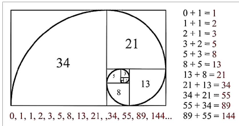
Рис.113. Числовой ряд Фибоначчи
