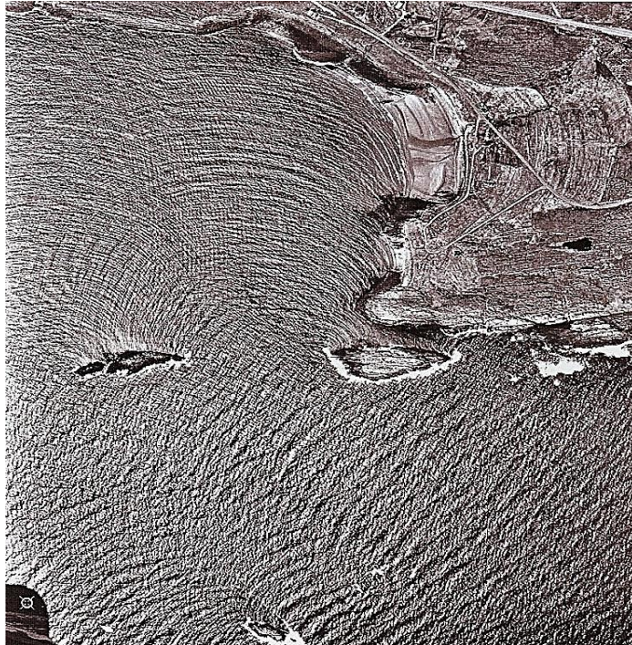
Рис.35. На снимке с высоты хорошо заметны все проявления дифракции волн на поверхности воды.
