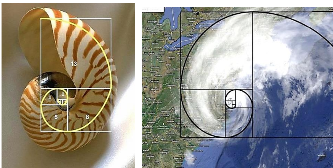
Рис.114
