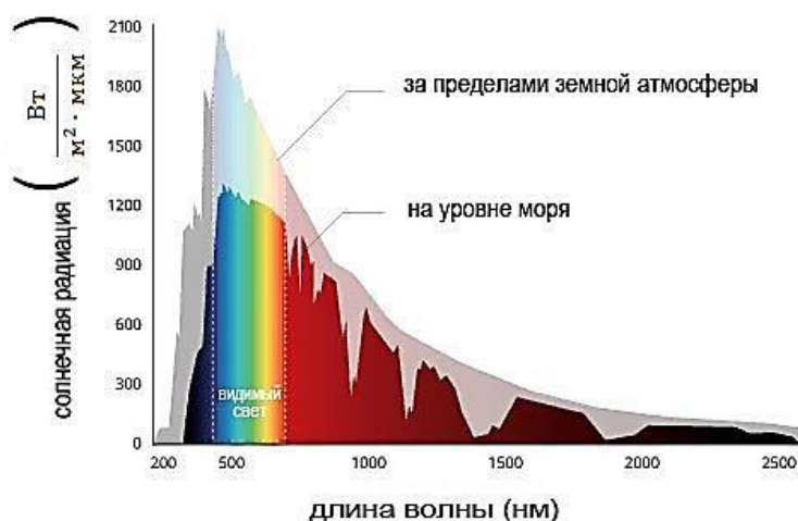
Рис.31. Солнце по разному выглядит в разных диапазонах.
