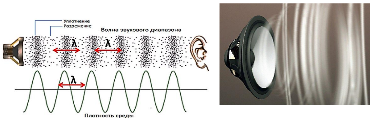
Рис.16. Источник, волна и плотность среды в волне
