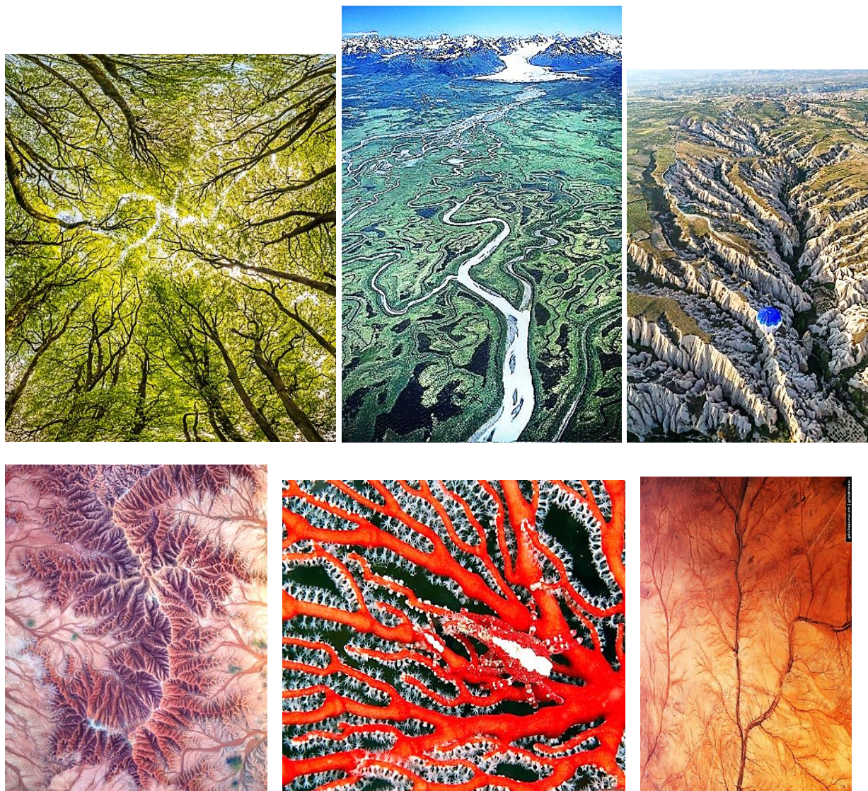
Рис. 111. Примеры природных фракталов
