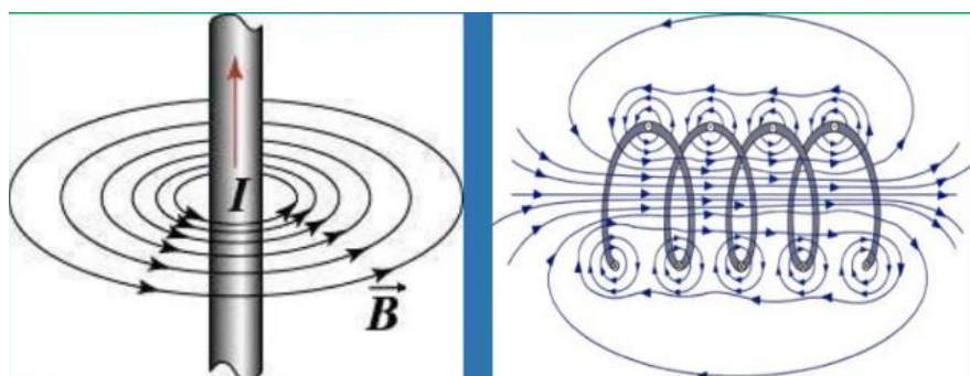
Рис.125. Форма магнитного поля прямого провода и провода, свёрнутого в спираль.
