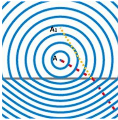
Рис.25. Так отличается истинное положение излучателя А от видимого А 1 при наблюдении из более плотной среды.
