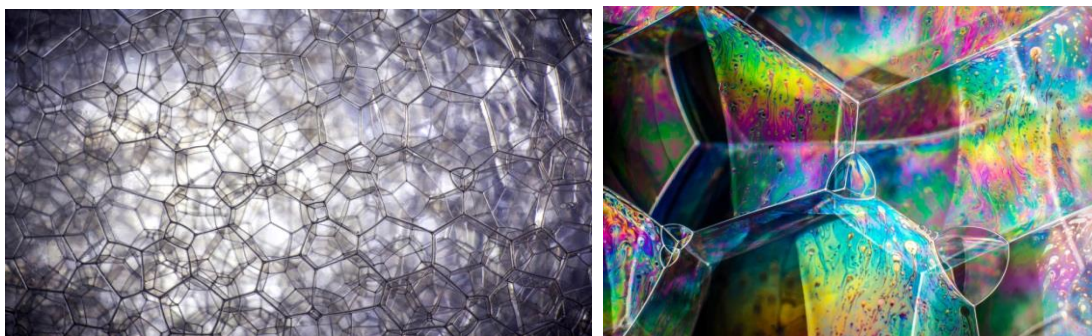
Рис.1. Пена
